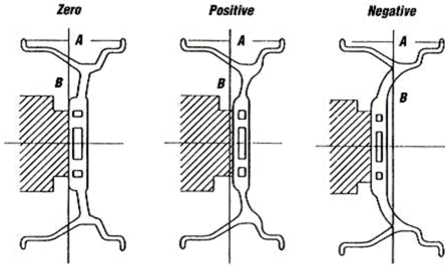
A = Rim Width B = Rim Centerline
